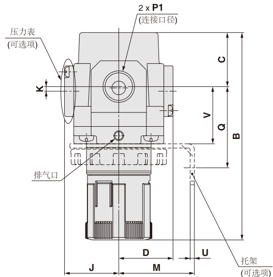
圆形压力表
