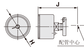
圆形压力表
